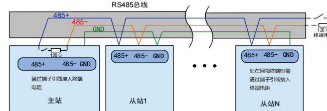
图 8 RS485 总线通信示意图
