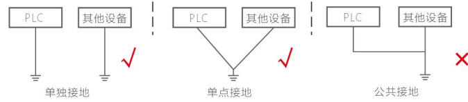
图1 接地类型图
