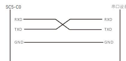
图 9 RS232 总线通信示意图
