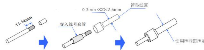
图 5 线缆制作示意图
