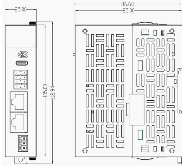
图 3 SC5-C0 产品外观尺寸图 (单位: mm)
