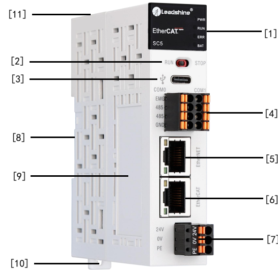
图2 SC5-C0 系列产品外部接口
